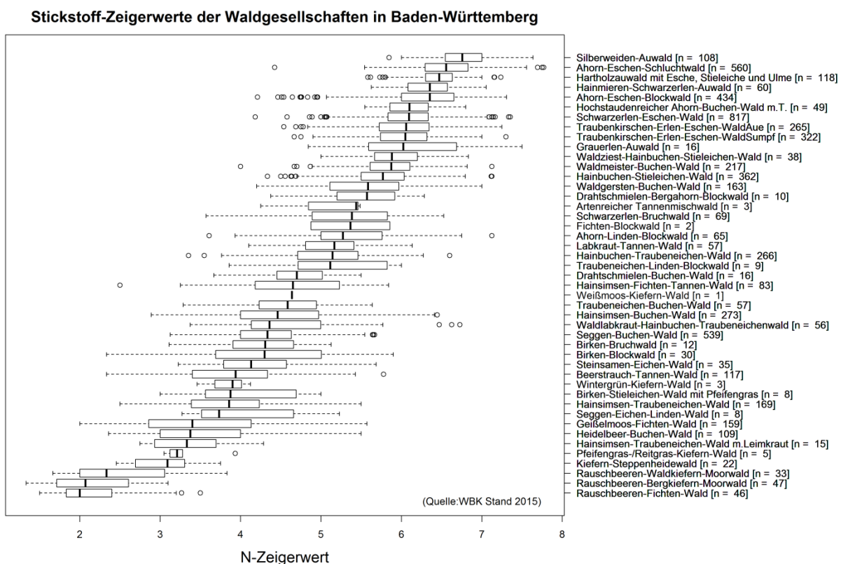
Abbildung 3-1: Mittlere Stickstoffzeigerwerte der Waldgesellschaften in Baden-Württemberg, basierend auf den ungewichteten Ellenberg-Stickstoffwerten der Gefäßpflanzen in der Bodenvegetation. [n = ] gibt die Anzahl der zugeordneten Biotope an.
