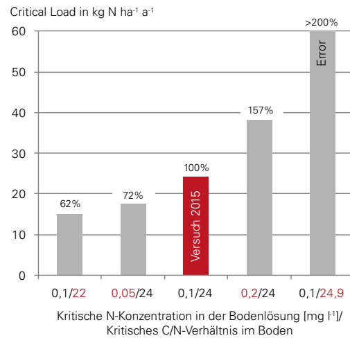
Abbildung 1-2: Bedeutung von zwei Eingangsgrößen für die Höhe der berechneten Critical Loads für eine ausgewählte Pflanzengesellschaft bei versuchsweiser Anwendung im Jahr 2015 mit der (damals) gültigen Formelsammlung (StickstoffBW 2014 und 2016)
